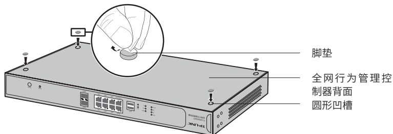
图2-3 桌面安装示意图
